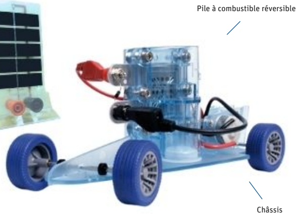
Châssis
